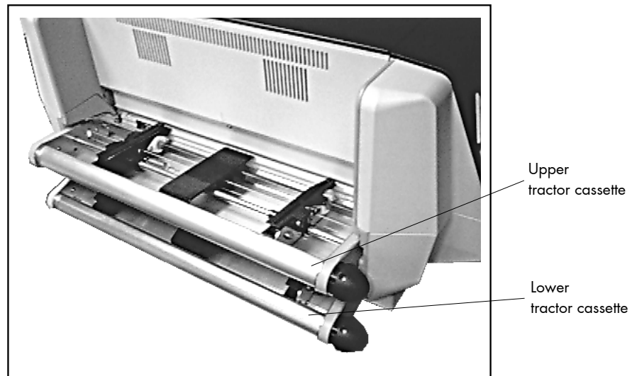
Fig. 4.1.1.a Tractor cassette position
